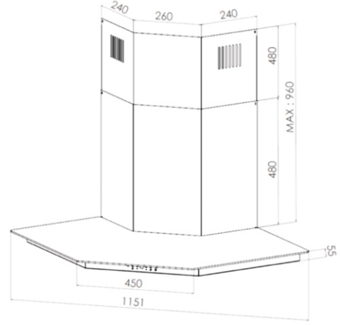
90'LİK KÖŞE MODEL DAVLUMBAZ MONTAJ ÖLÇÜSÜ
